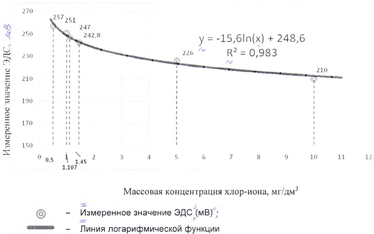
Рисунок В.1 — Зависимость ЭДС (мВ) от концентрации хлор-иона (мг/дм 3 )
